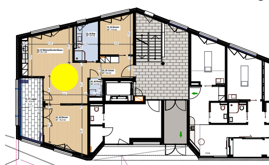
Grundriss EG Haus 2a „Ahorn“
