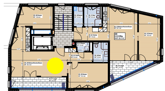
Grundriss 2. OG Haus 2 „Linde“
