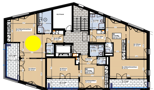
Grundriss 5. OG Haus 2a „Ahorn“
