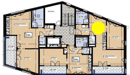
Grundriss 5. OG Haus 2a „Ahorn“
